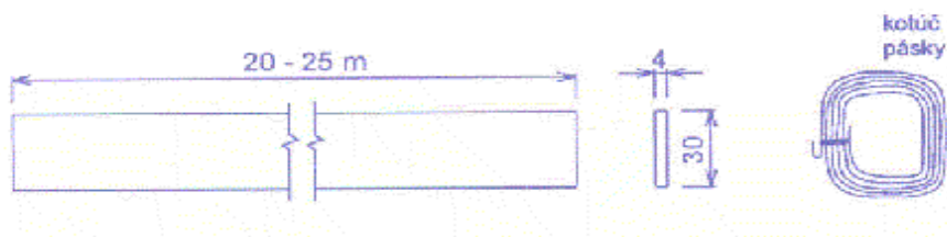
Obr.č.2: – Uzemňovacia páska 30 x 4 mm
